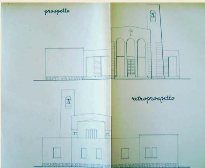
Fig. 6 - Progetto esecutivo della chiesa di Borgo Schisina.
